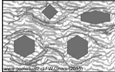
Figura: Textura porfiroblástica
